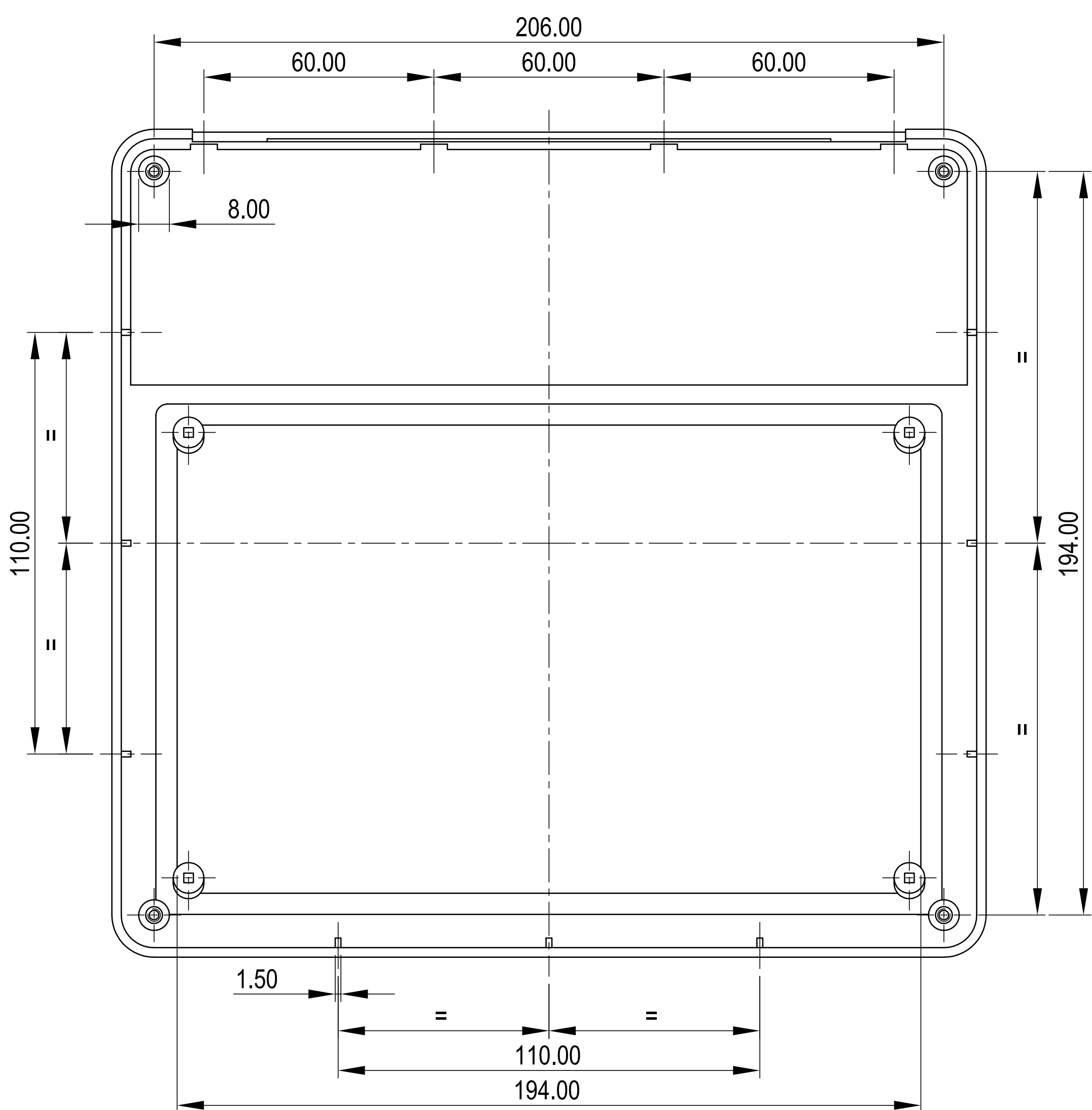
Oberteil Aussenansicht Top part Outside view
