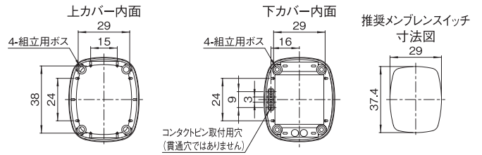
OAB-046□□-WT (上カバー凹部有)
