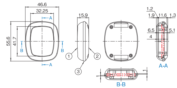
OAB-046□□-WT (上カバー凹部有)
