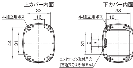
OAA-056□□-WT (上カバー凹部なし)
