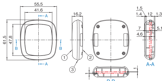
OAB-056□□-WT (上カバー凹部有)
