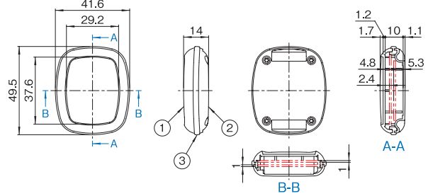
OAB-041□□-WT (上カバー凹部有)
