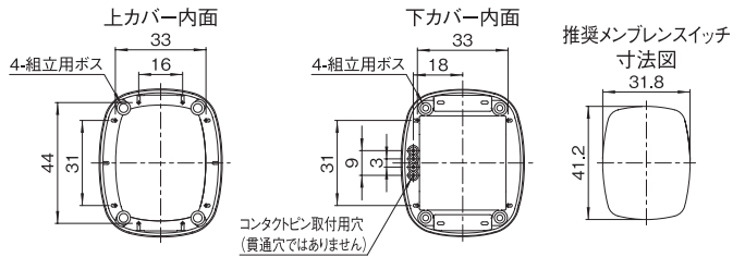
OAB-056□□-WT (上カバー凹部有)
