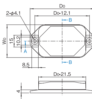
OJD-□□□□-□□ (長方形フランジ付)
