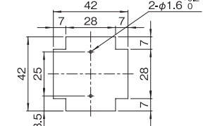
OJA/OJB-55□□-□□ 推奨PCBサイズ (上カバー/下カバー)
