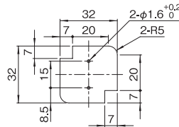
OJA/OJB-44□□-□□ 推奨PCBサイズ (上カバー/下カバー)
