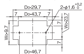
OJD-□□□□-□□ 推奨PCBサイズ (上カバー/下カバー)
