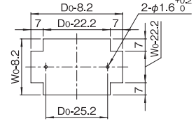
OJC-□□□□-□□ 推奨PCBサイズ (上カバー/下カバー)
