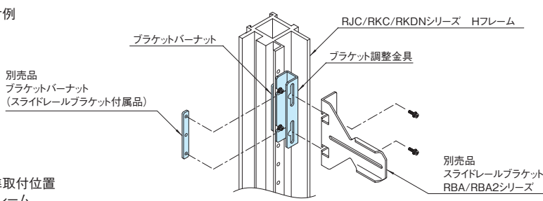
取付例
