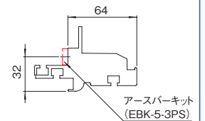
D部詳細
