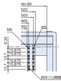
C部詳細
