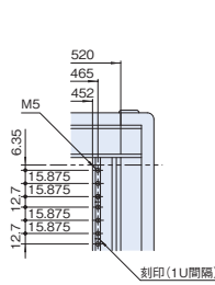
B部詳細
