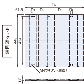
NPWS-44□□-N□
