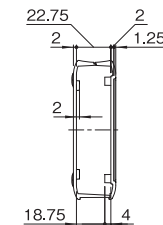
A-A (VLA-1509-□M)
