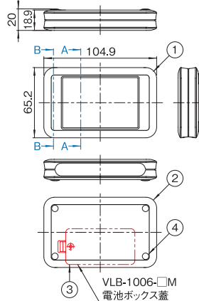
B-B (VLA-1006-□M)
