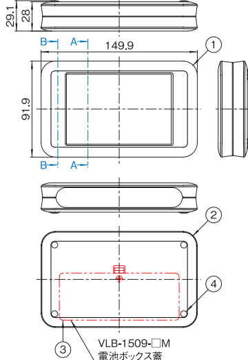
B-B (VLA-1509-□M)
