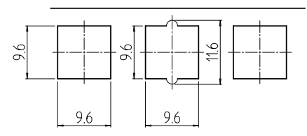
A部詳細 (1 : 1)
