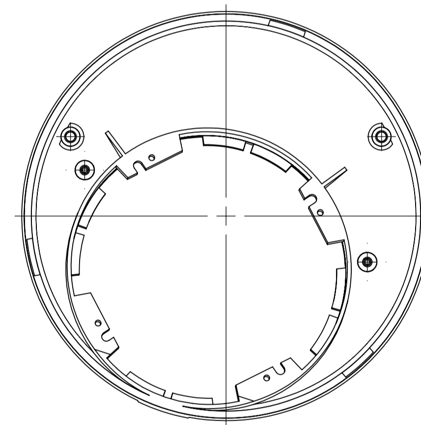
Unterteil-Innenansicht Bottom-Part-Inside-View
