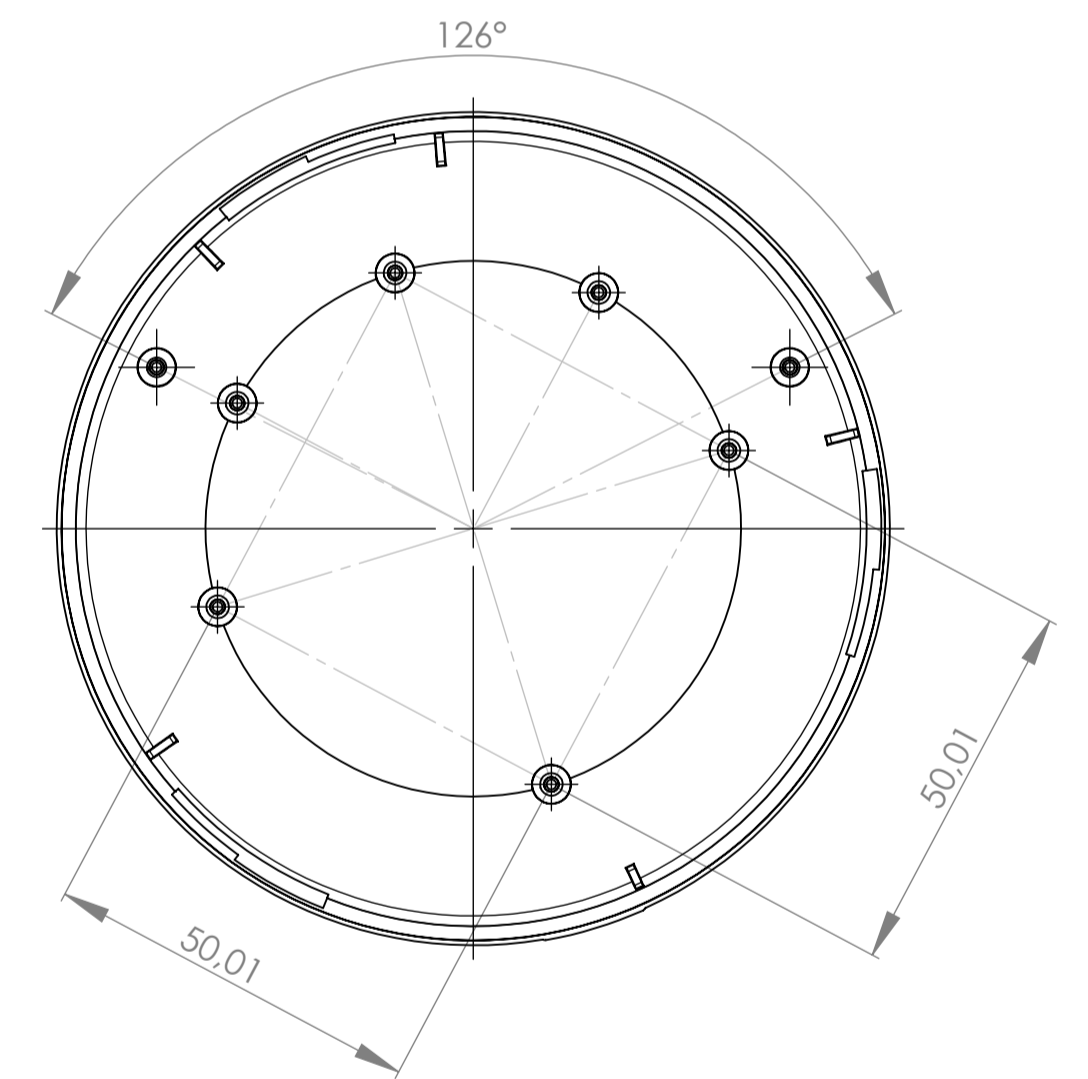
Oberteil-Innenansicht Top-Part-Inside-View
