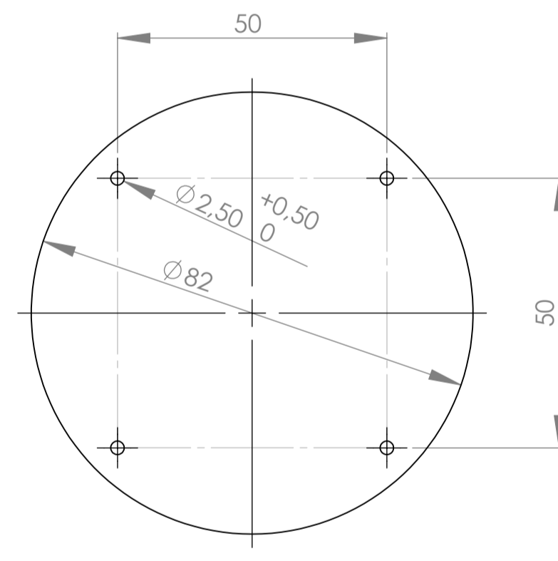
SCHNITT C-C
