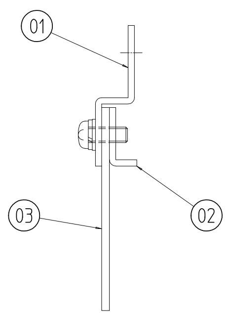
A-A (1 : 1)
