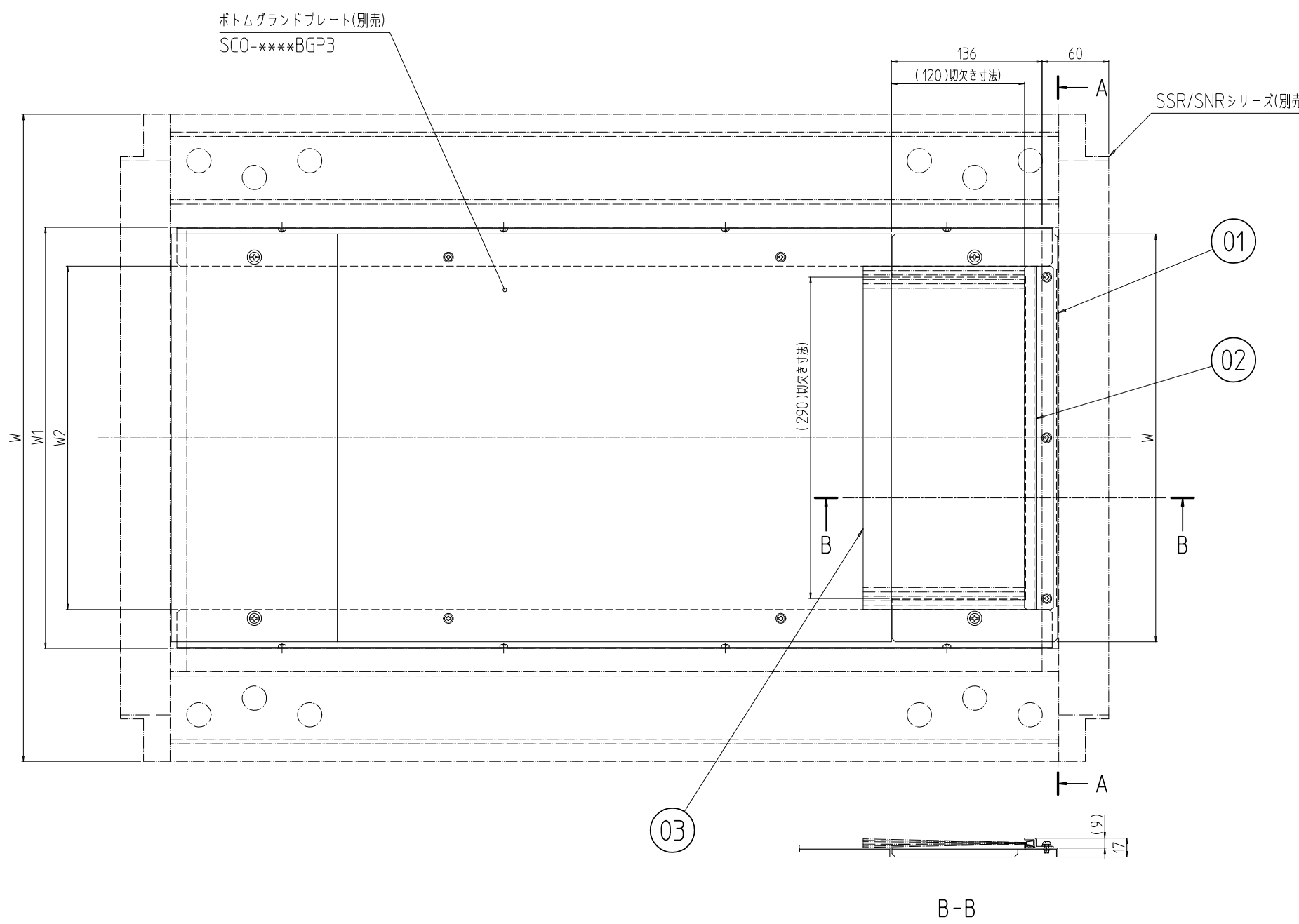
ラック実装図 内側から底面を見た図
