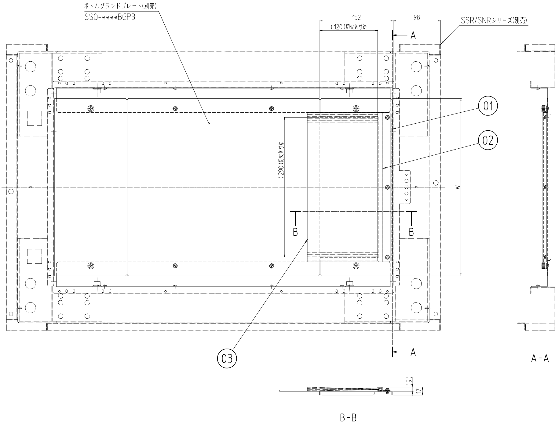
ラック実装図 内側から底面を見た図
