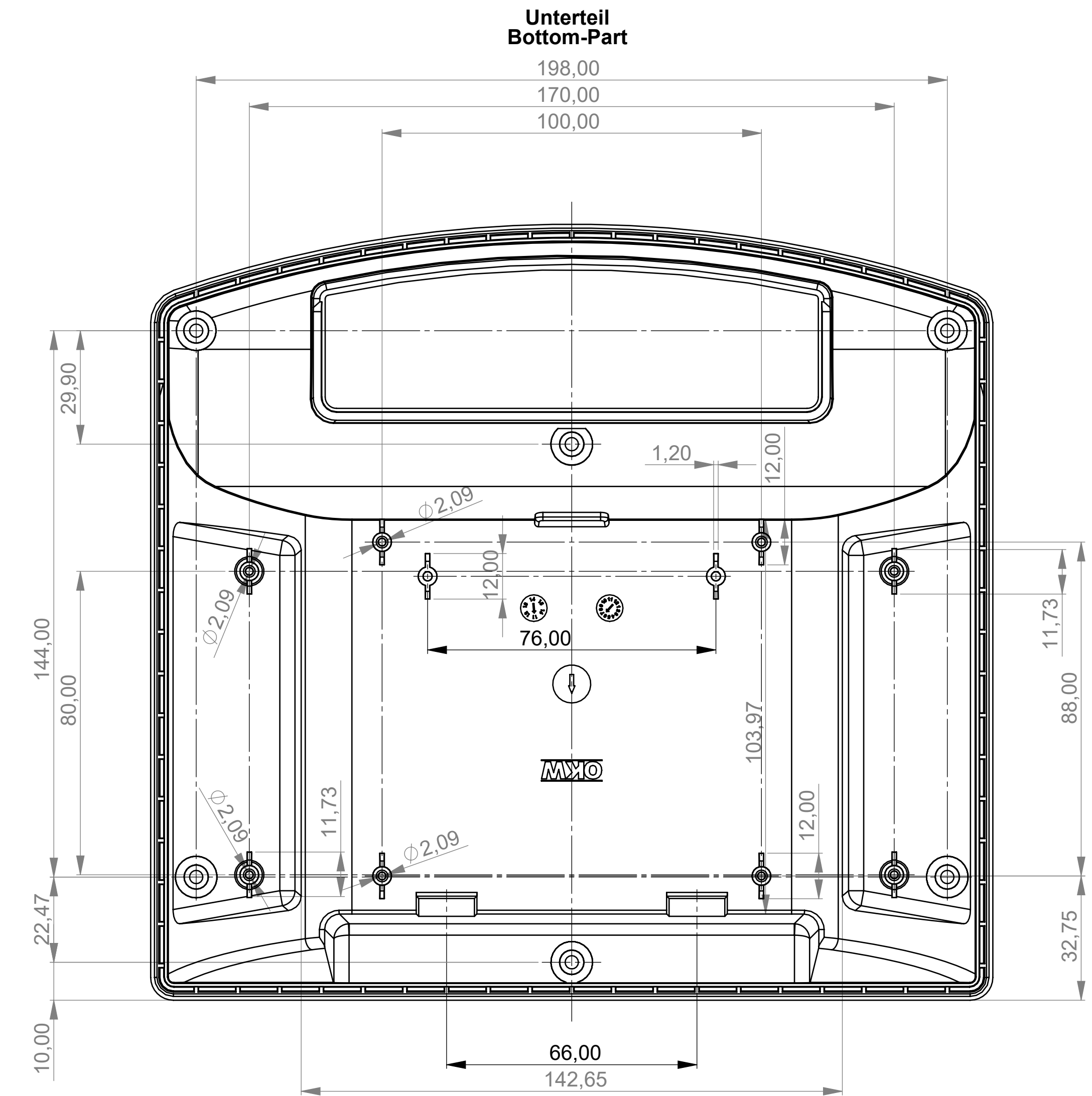
Platine Unterteil P C B Bottom Part
