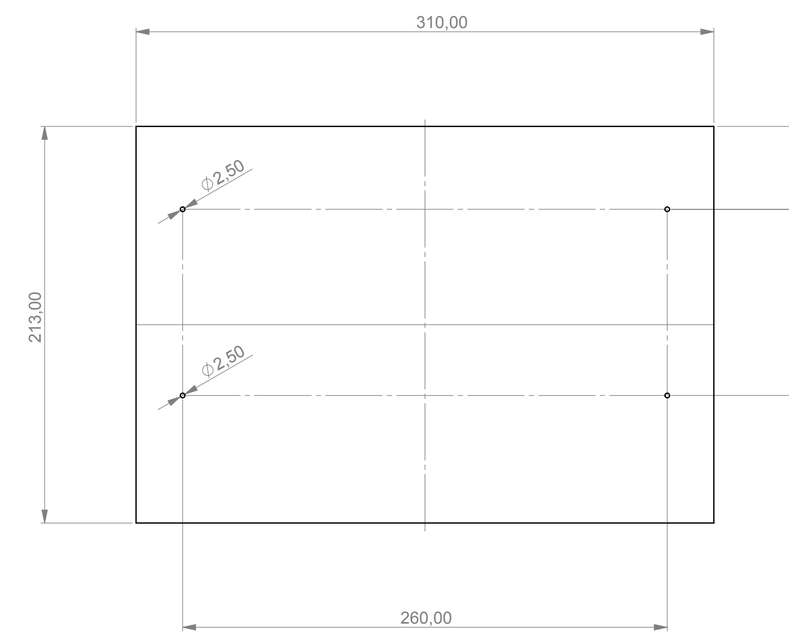
Platine Unterteil P C B Bottom Part
