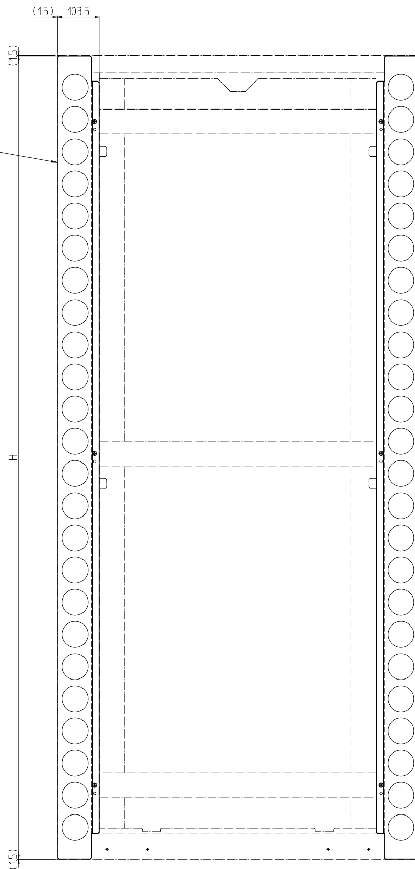
側面図 (1 : 10)
