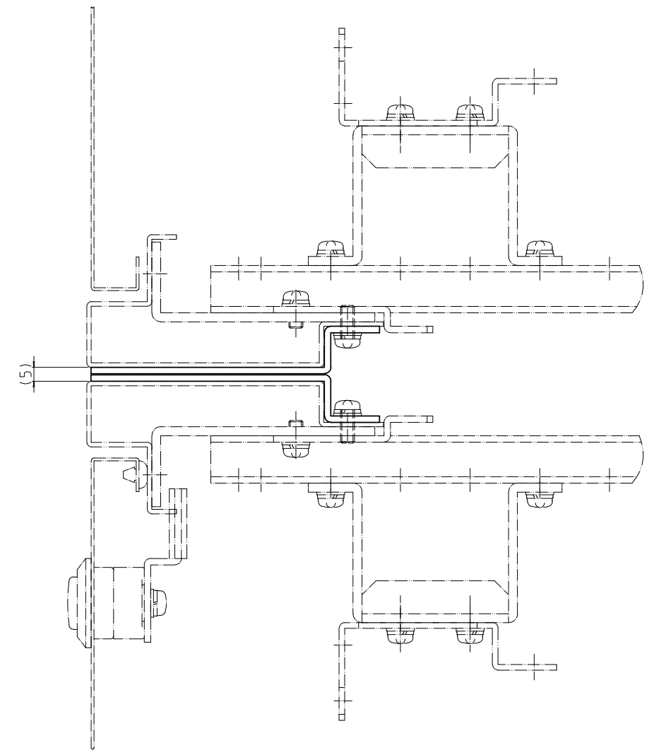
水平断面図
