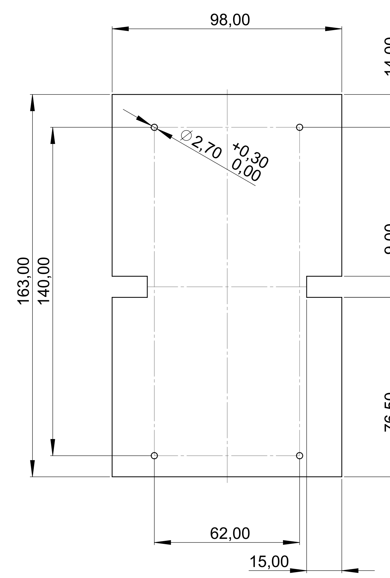
Platine Unterteil P C B Bottom Part
