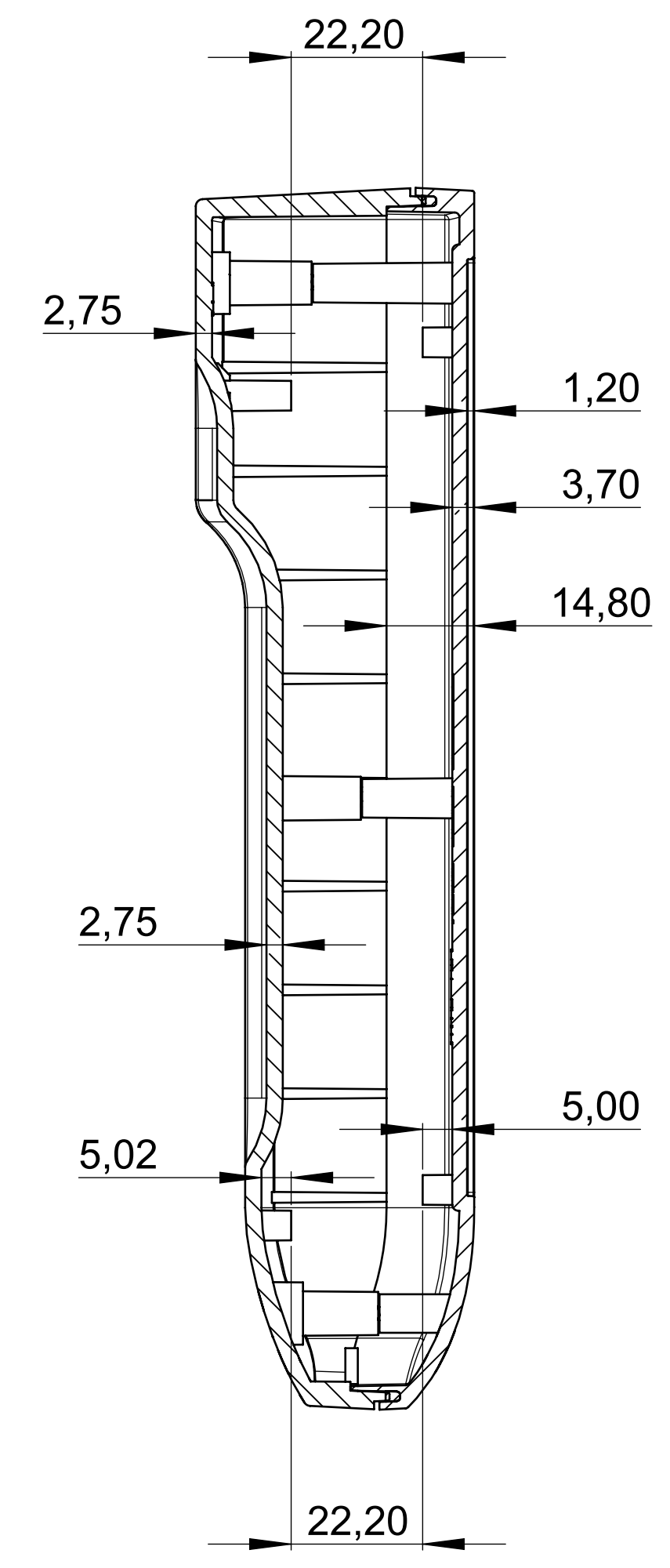
Schnitt A-A Section A-A
