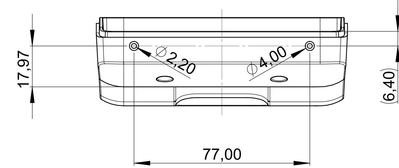
Unterteil Bottom-Part
