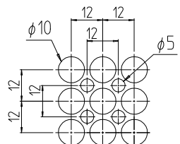
パンチング部詳細 (1 : 2) 開口率 約68%
