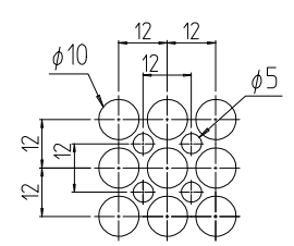
パンチング部詳細 (1 : 2) 開口率 約68%
