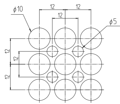
パンチング部詳細 (1:1) 開口率 約68%
