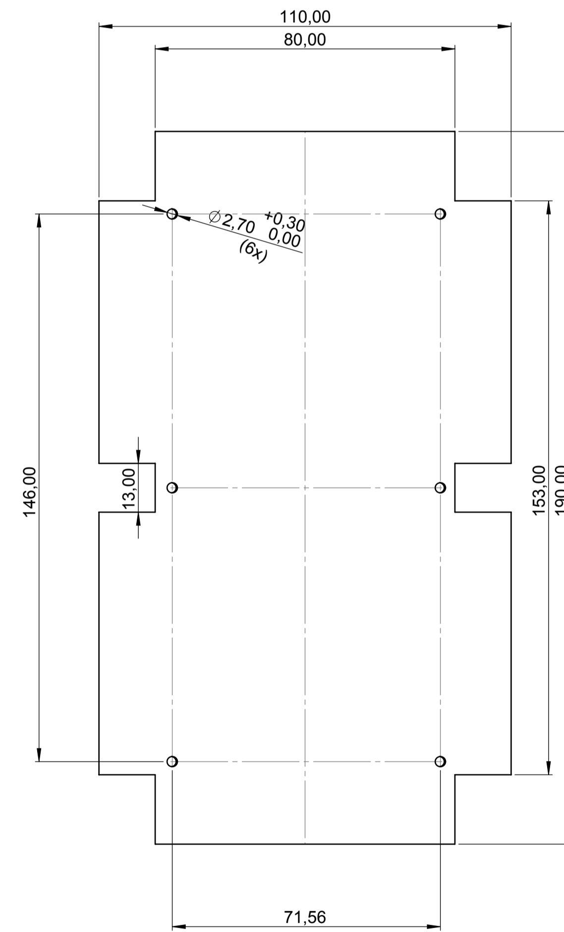
Platine Oberteil P C B Top Part
