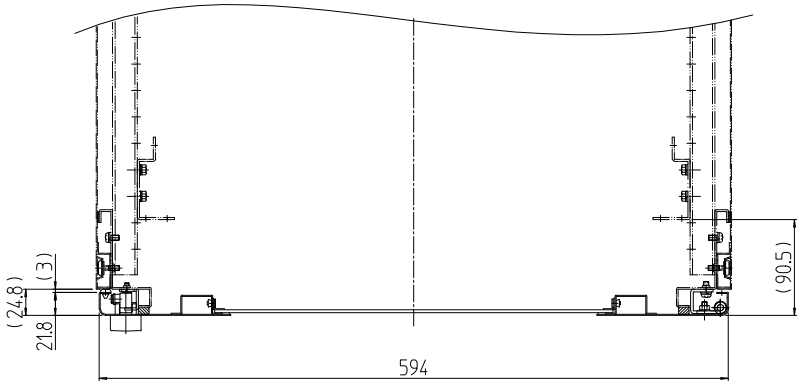
A-A (1 : 7)
