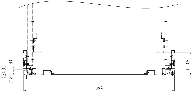
A-A (1 : 7)
