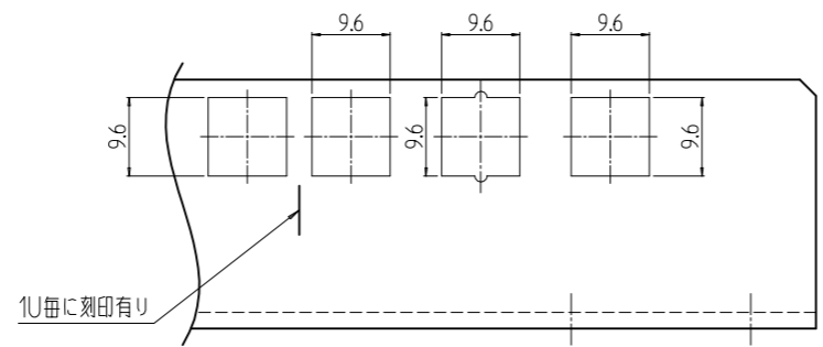
A部詳細 (1:1)
