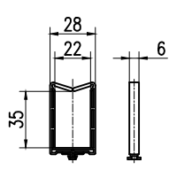
コードガイド寸法図
