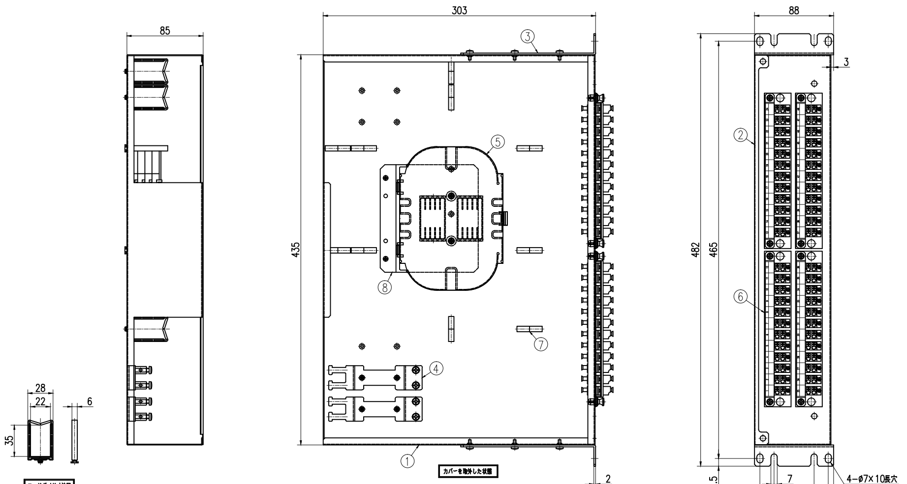
コードガイド寸法図
