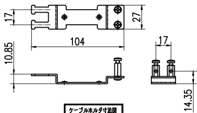
ケーブルホルダ寸法図
