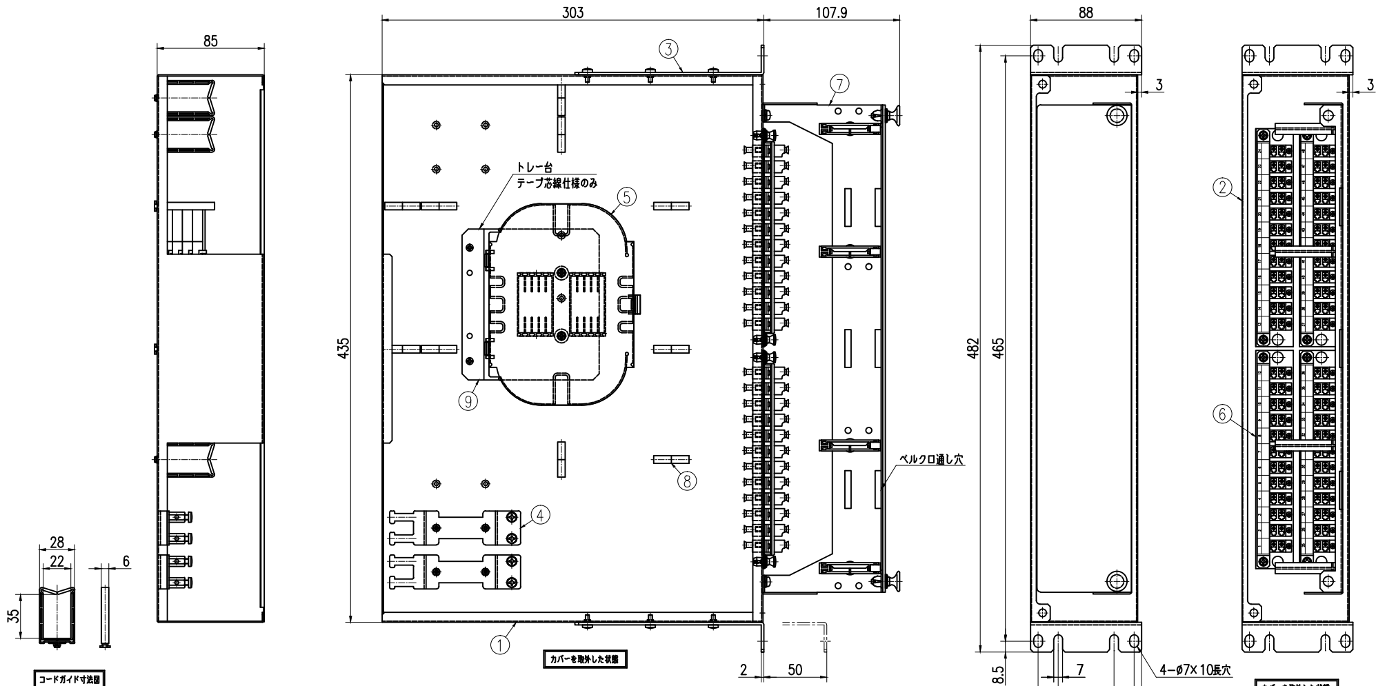
コードガイド寸法図
