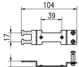
ケーブルクランプ斜め取付位置
