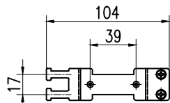
ケーブルクランプ斜め取付位置
