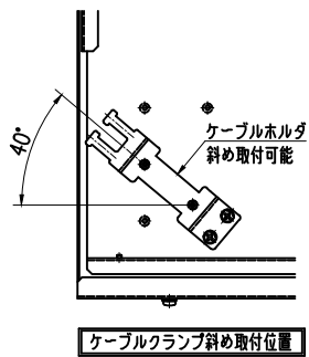
ケーブルクランプ斜め取付位置
