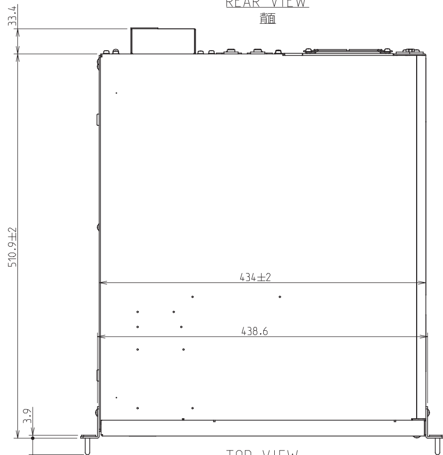
TOP VIEW 平面
