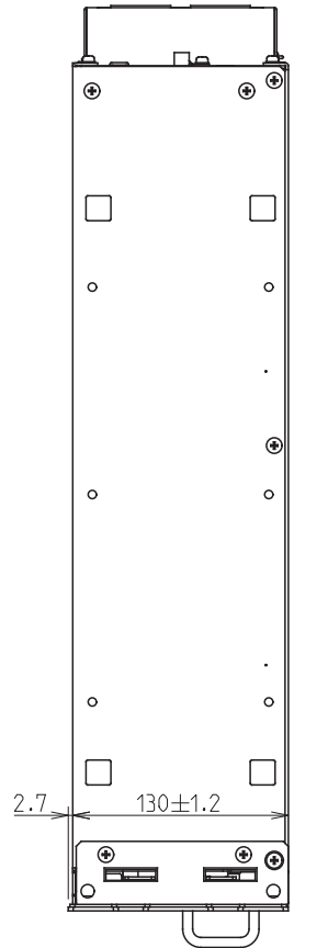
LEFT SIDE VIEW 左側面
