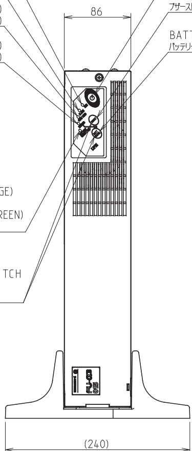
FRONT VIEW 正面
