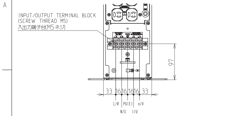
INSIDE VIEW OF TB COVER TBカバー内部
