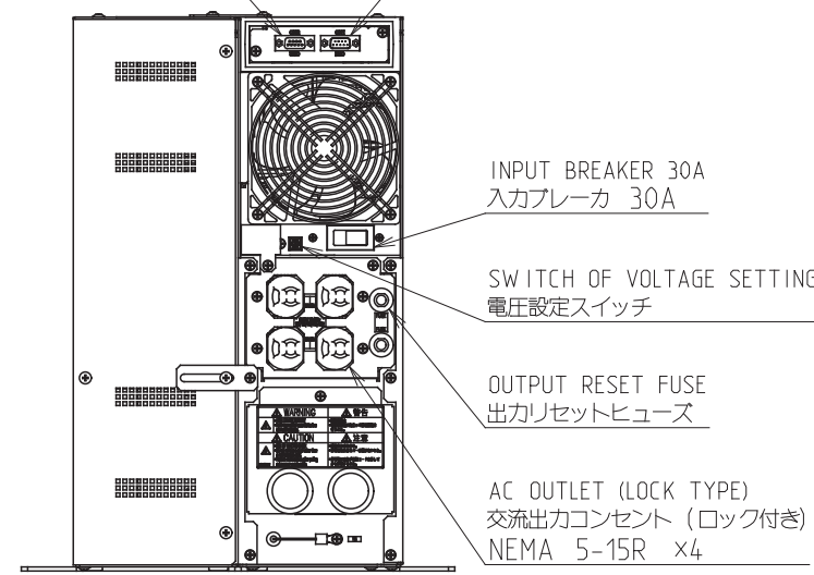
REAR VIEW 背面
