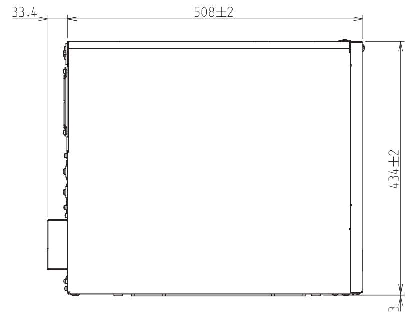
LEFT SIDE VIEW 左側面
