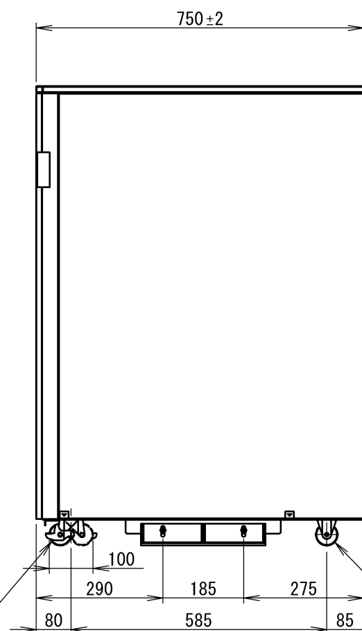
RIGHT SIDE VIEW 右側面
