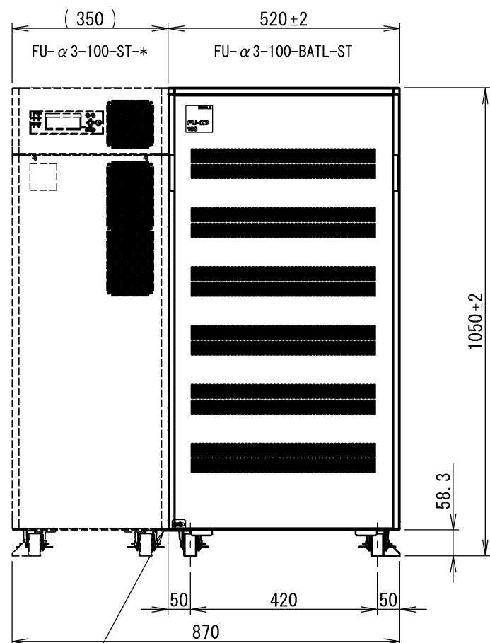
FRONT VIEW 正面
