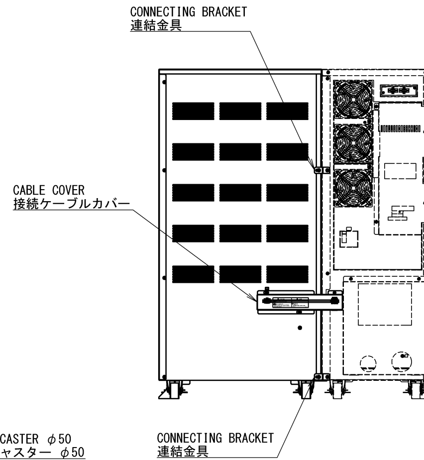
REAR VIEW 背面
