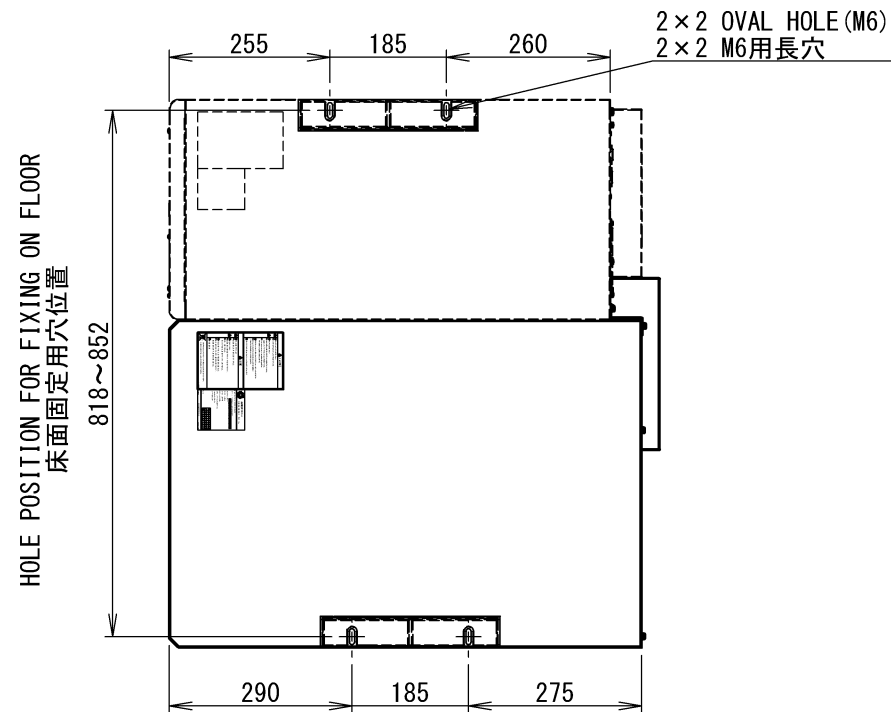
TOP VIEW 平面
