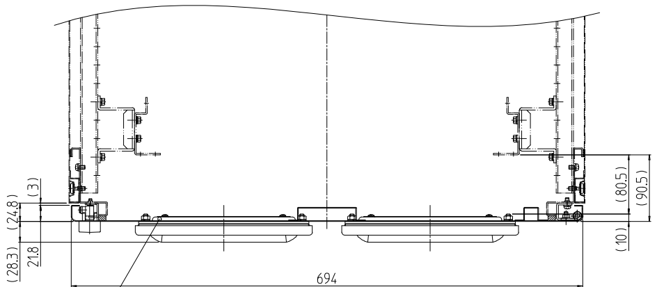
(内部) 08 09 A-A (1:7)
