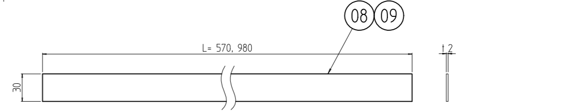
アングル用ゴム詳細 (1 : 4)
