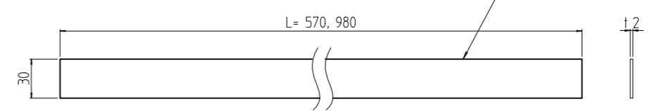
アングル用ゴム詳細 (1:4)
