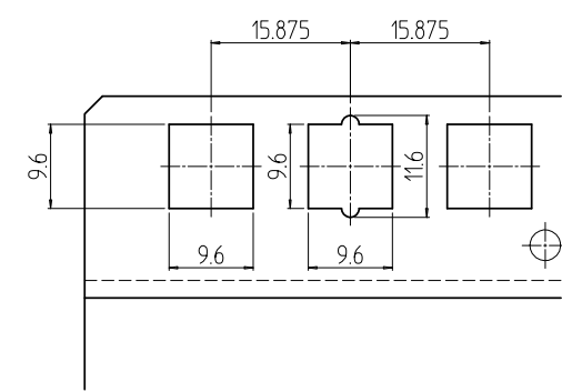
A部詳細 (1 : 1)
