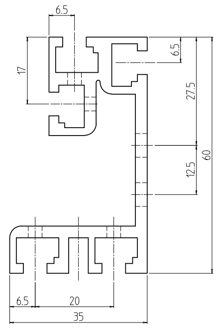
A-A (1 : 1)
