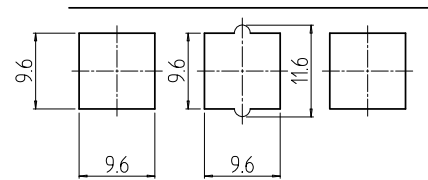
A部詳細 (1 : 1)
