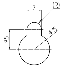
A穴詳細 (1:1)
