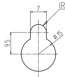
A穴詳細 (1 : 1)
