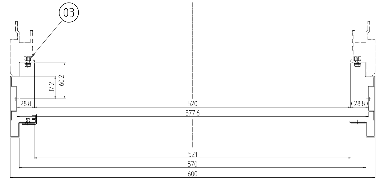
A-A (1 : 4)
