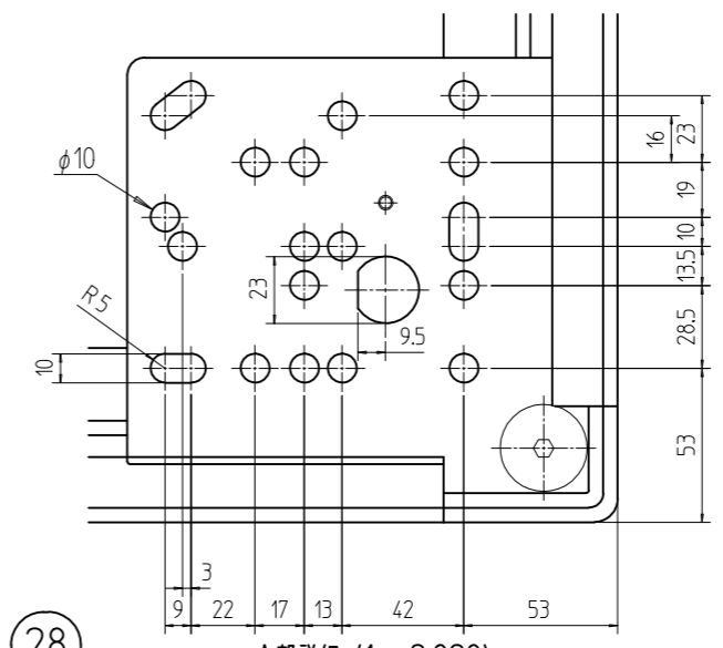
A部詳細 (1 : 2.828)
