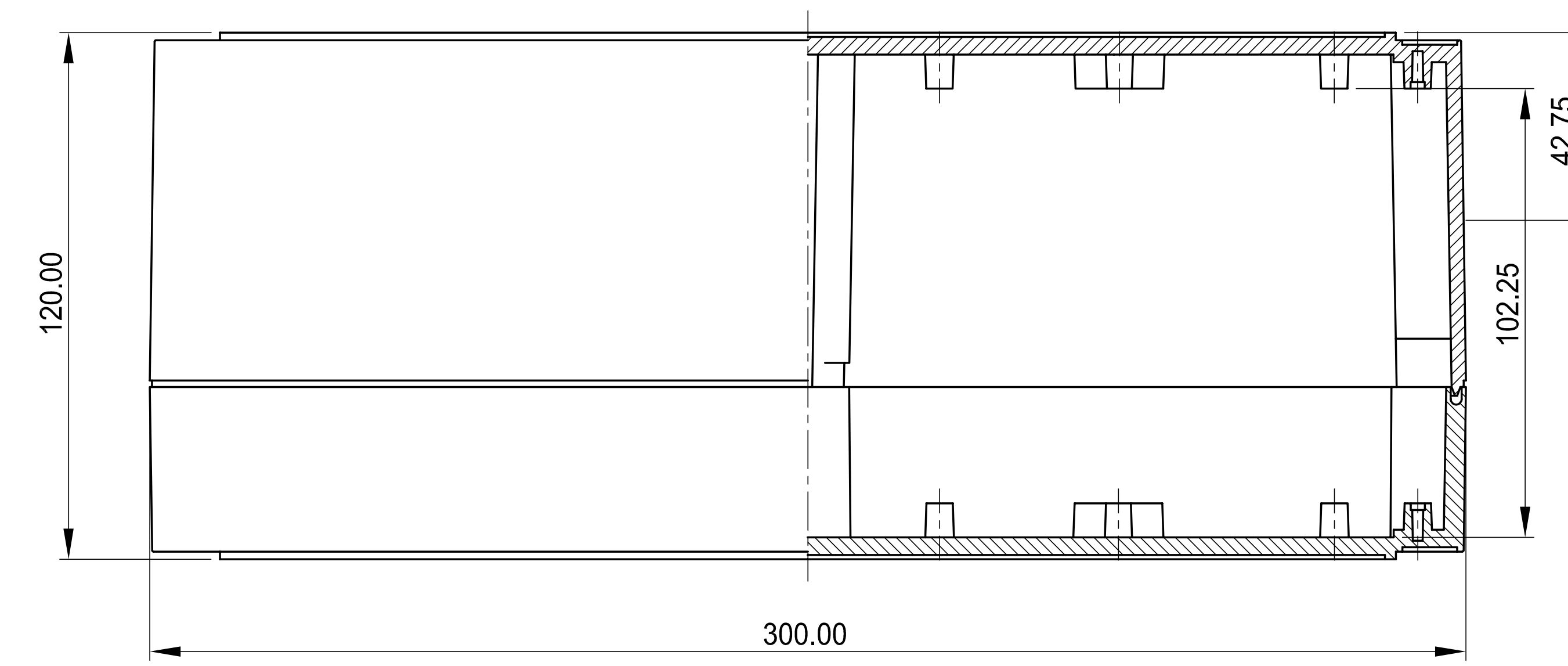
Schnitt A-A section
