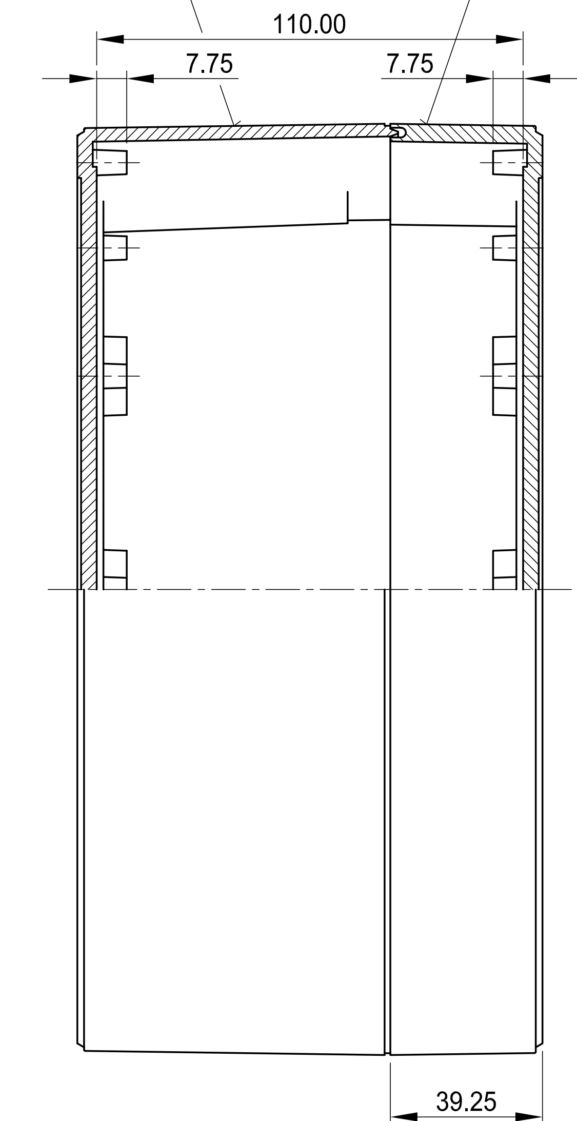
Schnitt B-B section
