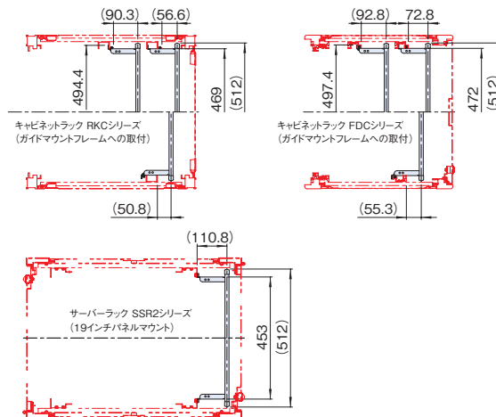
取付例
