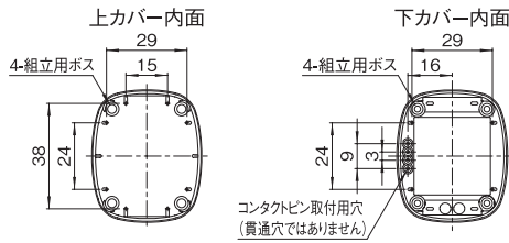
OAA-046□□-WT (上カバー凹部なし)
