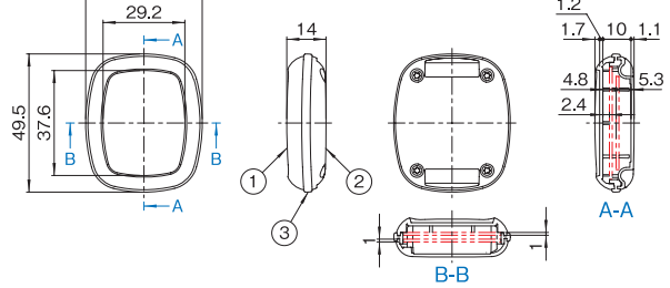
推奨メンブレンスイッチ 寸法図
