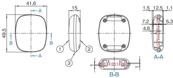
OAA-041□□-WT (上カバー凹部なし)
