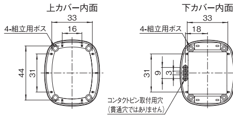
OAB-056□□-WT (上カバー凹部有)
