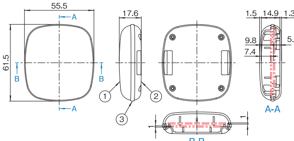
OAA-056□□-WT (上カバー凹部なし)
