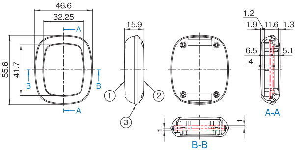
推奨メンブレンスイッチ 寸法図
