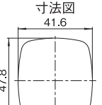
推奨メンブレンスイッチ 寸法図
