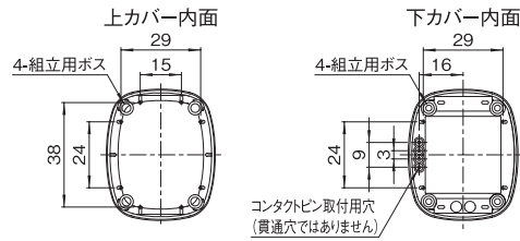
OAB-046□□-WT (上カバー凹部有)
