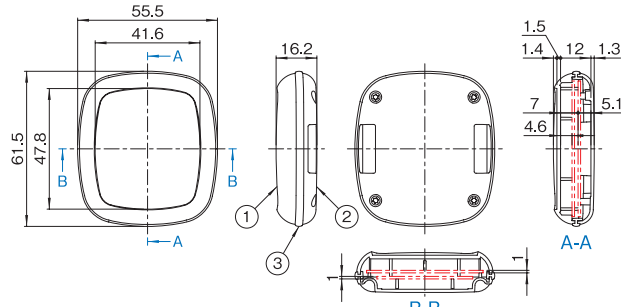
OAB-056□□-WT (上カバー凹部有)
