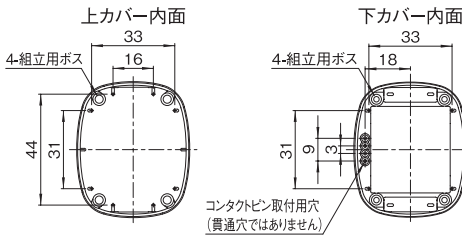
OAA-056□□-WT (上カバー凹部なし)
