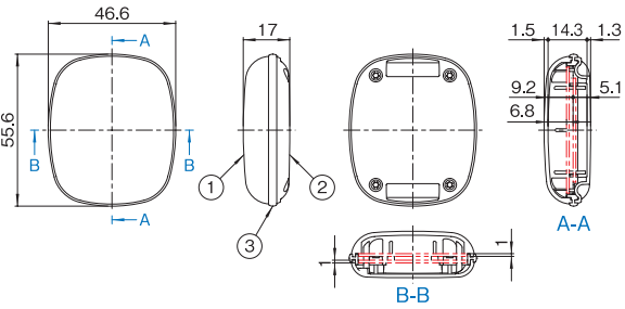
OAA-046□□-WT (上カバー凹部なし)
