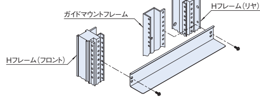
A部詳細
