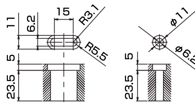
本体取付穴寸法
